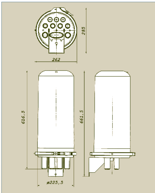
Schemat budowy mufy liniowej SEC 23
